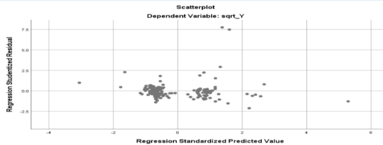
Ganbar 2. Uji Heteroskedastisitas
