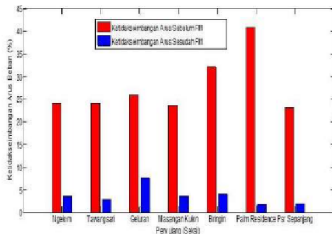
Gambar 10. Perbandingan Nilai Rata-Rata Ketidakseimbangan Arus Beban
