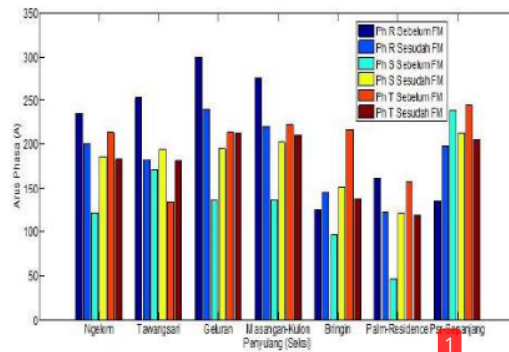
Gambar 9. Perbandingan Nilai Arus Beban Pada Fasa R, Fasa S, dan Fasa T
