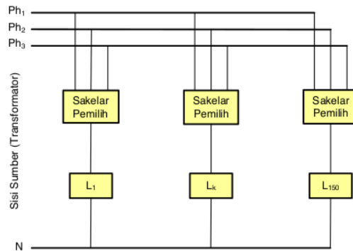
Gambar 6. Penyulang Saluran Distribusi dengan Sakelar Pemilih Fasa
