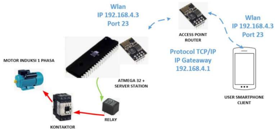
Gambar 3. Perencanaan Sistem Alat
