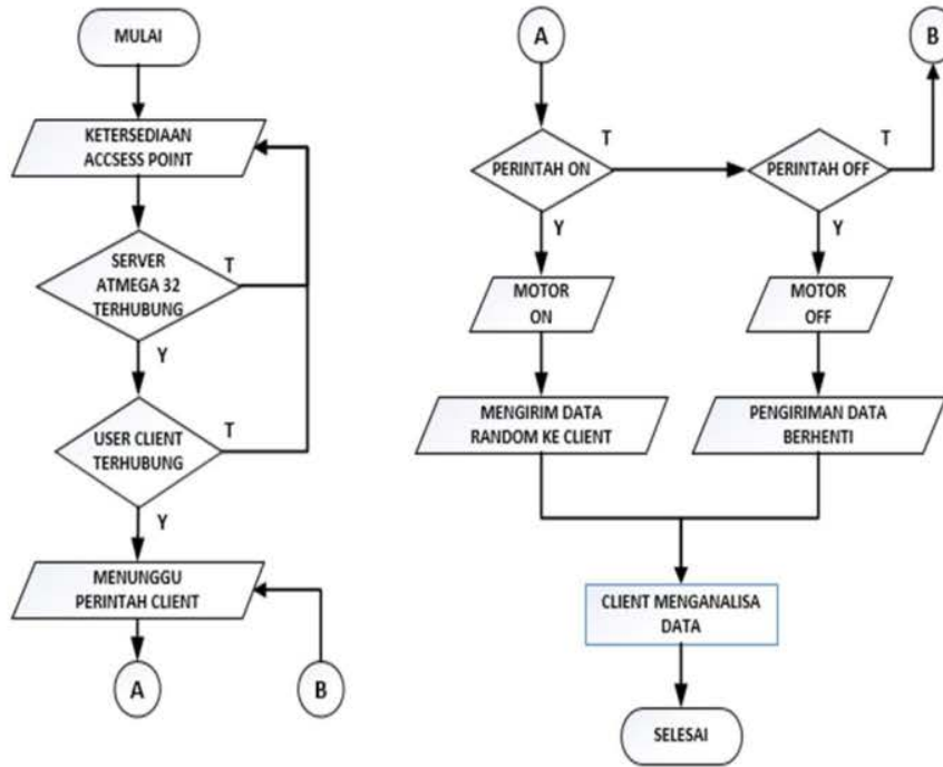
Gambar 4. Flowchart Sistem Kerja Alat
