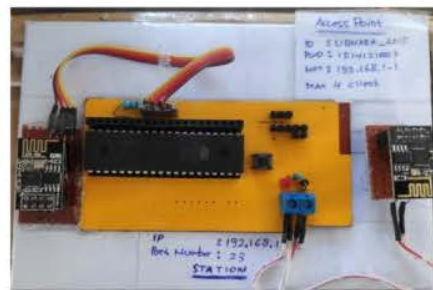
Gambar 8. Hasil Pembuatan Alat
