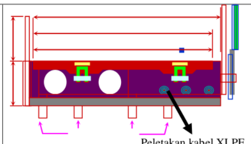
Gambar 2. Peletakan kabel disisi Jembatan Suramadu
