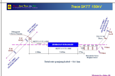
Gambar 4. SKTT menggunakan Kabel XLPE
