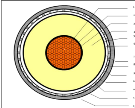
Gambar 6. Potongan melintang kabel isolasi XLPE 150 kV jenis single core . (Sumber: PT.PLN (Persero) P3B RJTB, 2010)
