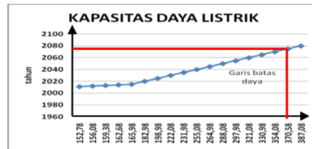
Gambar 7. Grafik Prediksi Kebutuhan Daya Listrik di Pulau Madura berdasarkan kapasitas Kabel 150 kV Isolasi XLPE Single Core yang Terpasang pada Jembatan Suramadu
