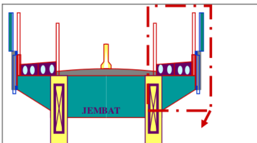
Gambar 1. Pemasangan kabel di Jembatan Suramadu
