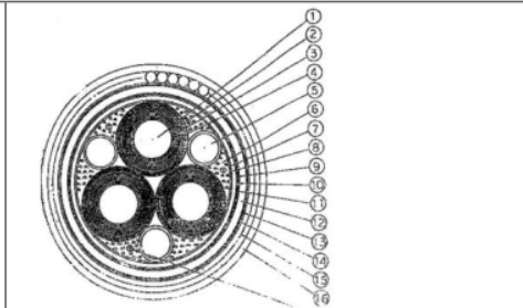
Gambar 7. Potongan melintang kabel isolasi minyak 150 kV jenis three core . (Sumber: Uppal, 1980)
