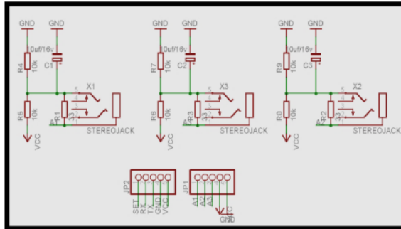
Gambar 7 : Skematik Rangkaian Sensor Arus
