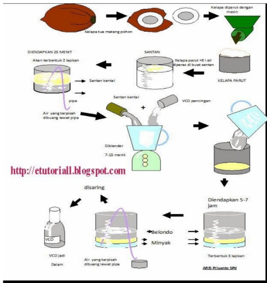
Gambar 3. Skema Pembuatan Minyak Kelapa
