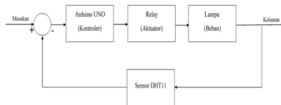
Gambar 3. Blok Diagram Sistem Mesin Penetas Telur
