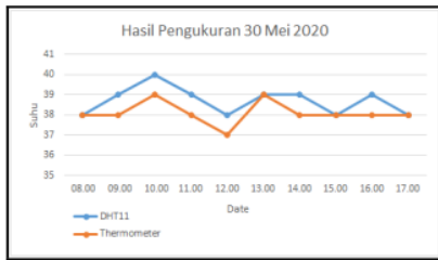
Gambar 7. Grafik Pengambilan Data Suhu Pertama
