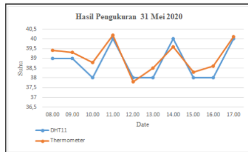
Gambar 9. Grafik Pengambilan Data Suhu Kedua
