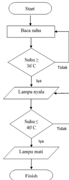
Gambar 4. Flowchart Cara Kerja Mesin Penetas Telur
