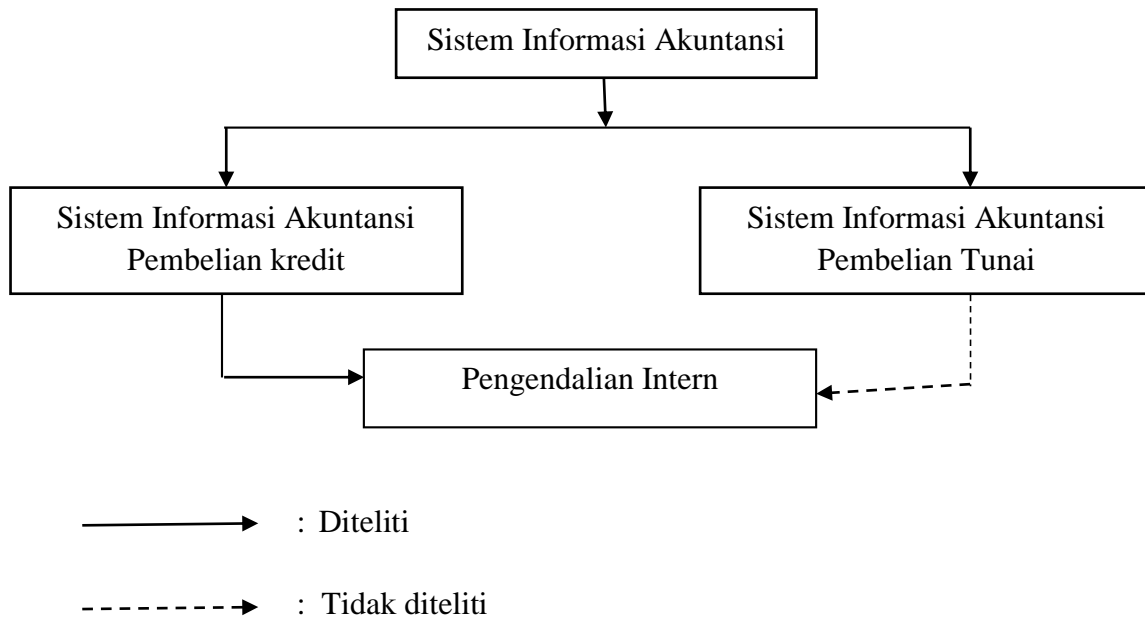
Gambar 1 Kerangka Konseptual
