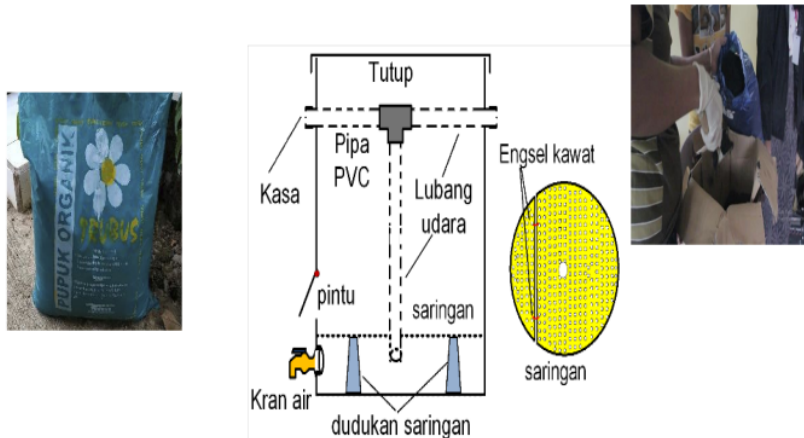
Gambar 2. Ember untuk pembuatan komposter
